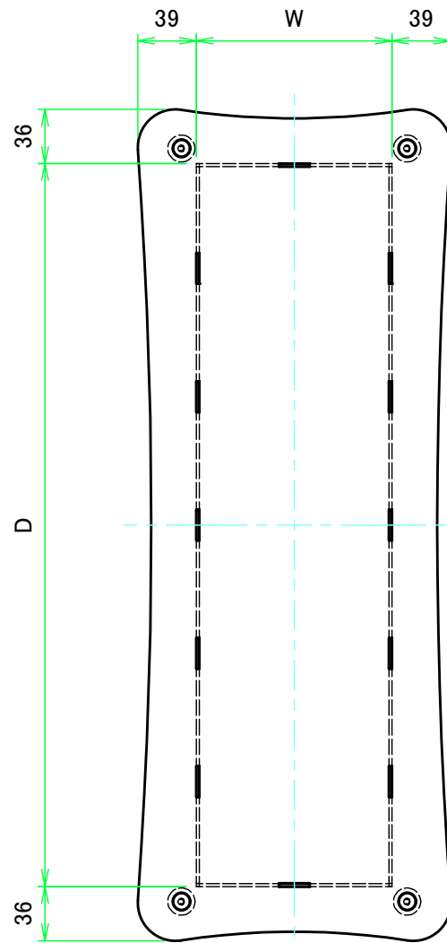
Wパネル1 / W panel 1
